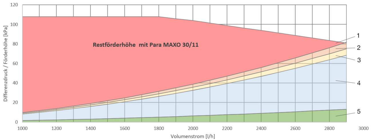
Wärmepumpe VampAir PRO 15 mit Anschlusset nach unten + Hydromodul: Umwälzpumpe: Para MAXO 30/11
