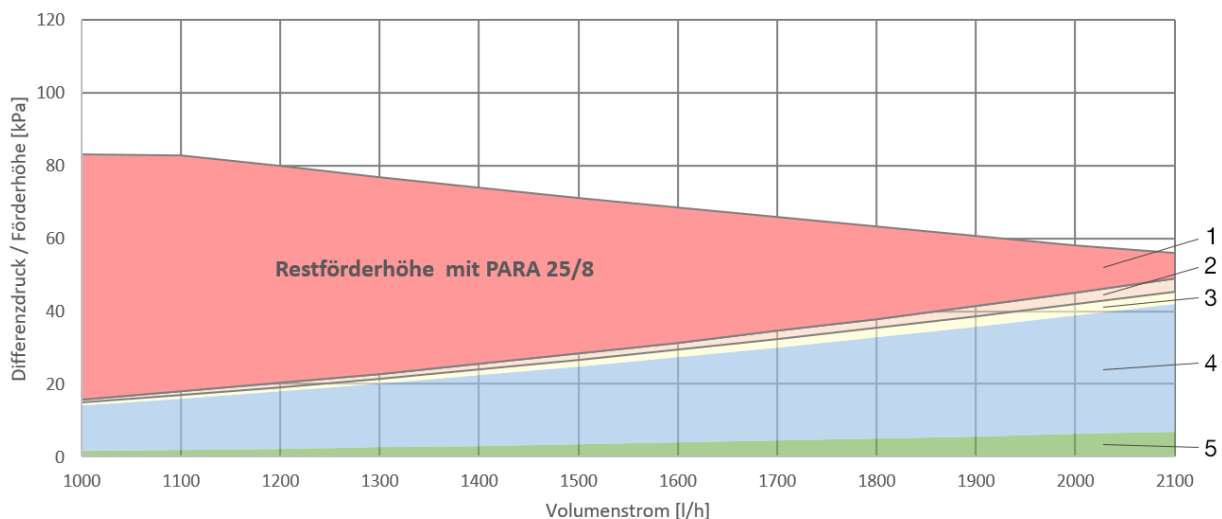
Wärmepumpe VampAir PRO 10 mit Anschlusset nach unten +Hydromodul Umwälzpumpe: PARA 25/8
