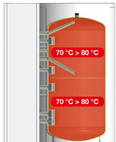
Schnittbild hydro tower PVmax
