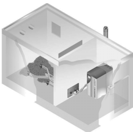
Pellets-Heizcontainer
