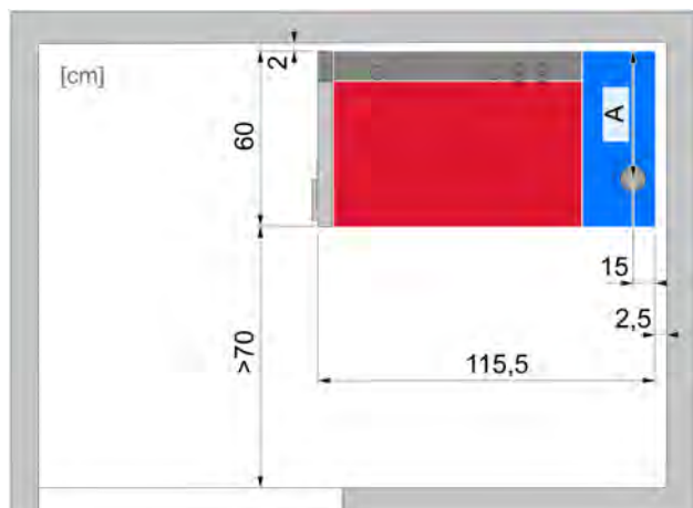
Kaminanschluss oben
