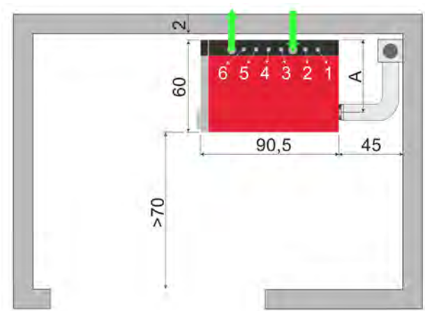
Kaminanschluss oben
