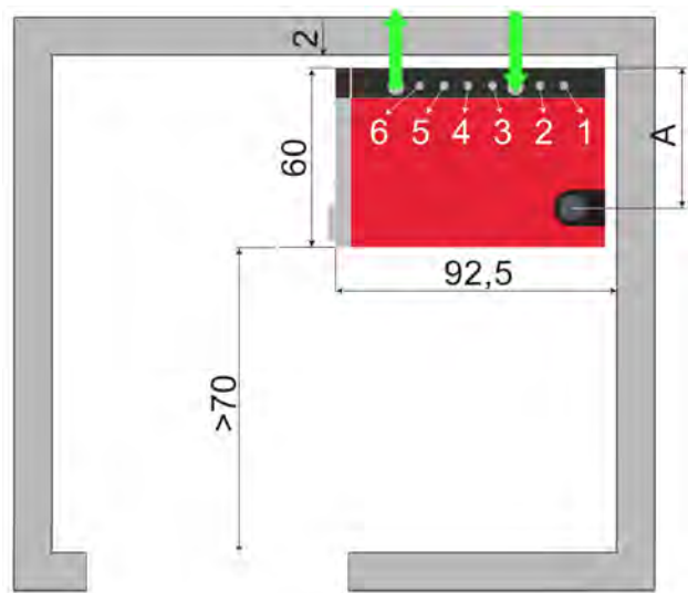
Kaminanschluss oben
