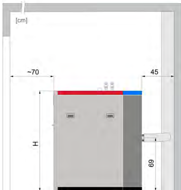
Kaminanschluss hinten
