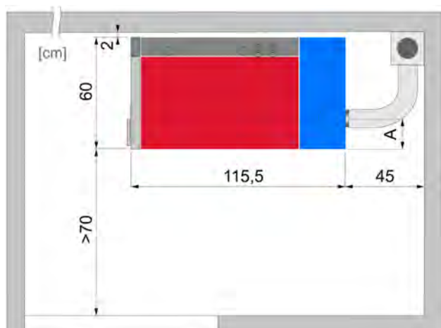
Kaminanschluss oben
