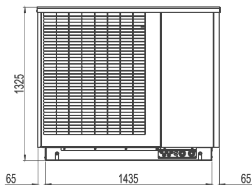
Ansicht hinten
