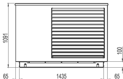
Ansicht vorne
