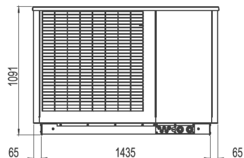
Ansicht hinten
