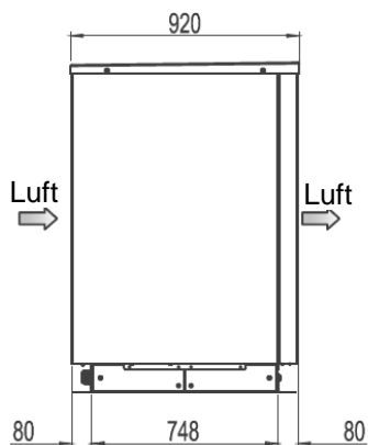
Ansicht Seite
