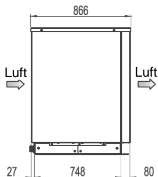
Ansicht Seite
