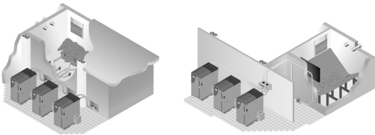
Kessel-Kaskadenlösung mit unterschiedlichem Lager-/Fördersystem
