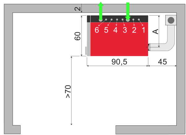
Kaminanschluss oben
