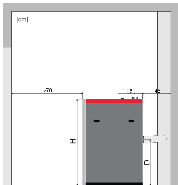
Kaminanschluss hinten
