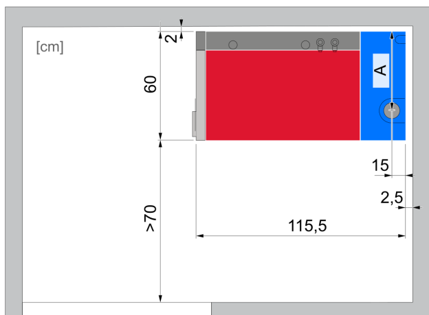
Kaminanschluss oben
