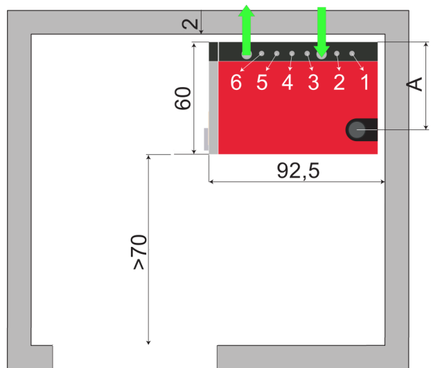
Kaminanschluss oben
