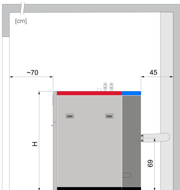
Kaminanschluss hinten
