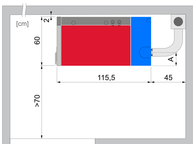
Kaminanschluss oben
