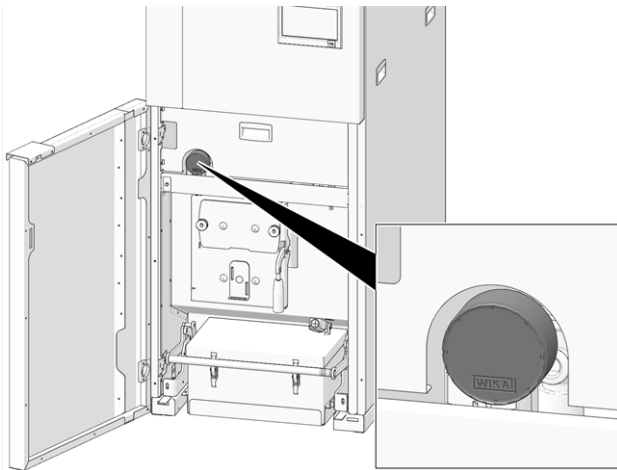
Abb. 2-51_Position des Manometers
